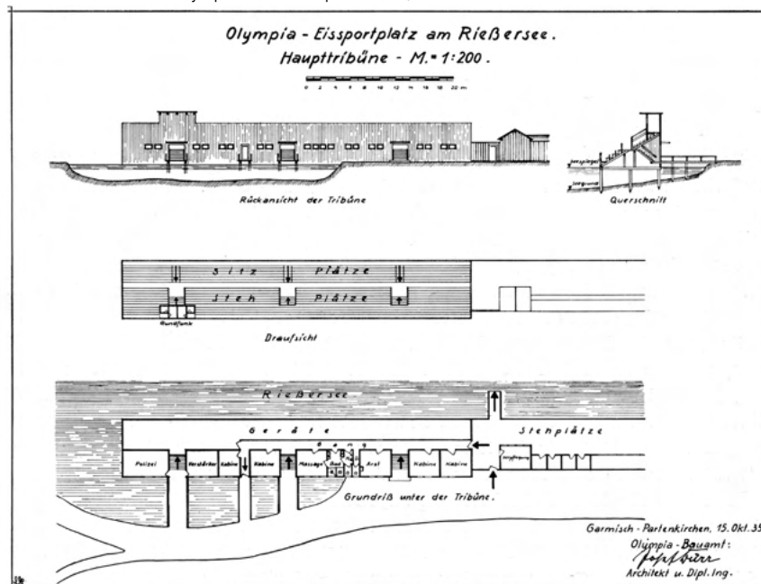
Ansicht und Grundriss der Haupttribüne Marktarchiv Garmisch-Partenkirchen
